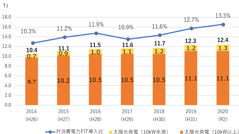
図 2-2-5 再エネ発電量(FIT)の推移
