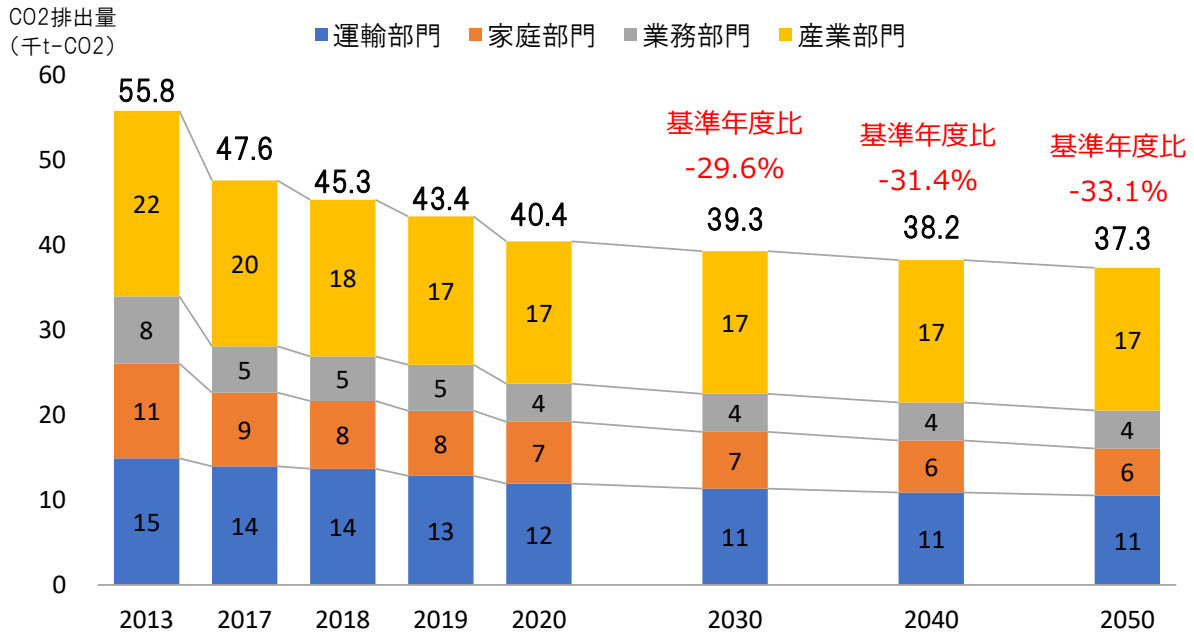
図 3-3-2 BAU 推計による将来時点のCO2排出量の推移
